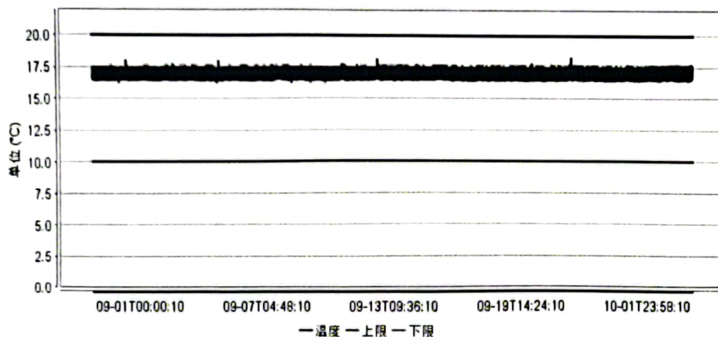
温度曲线图
