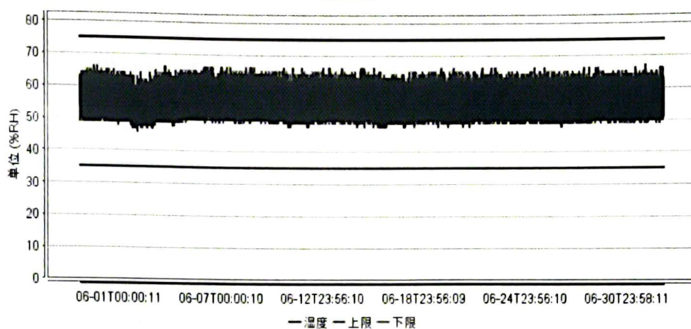
湿度曲线图
